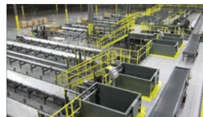
Despaletizadores semiautomáticos
